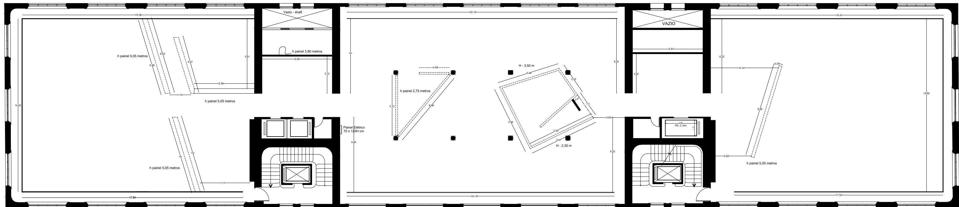
PLANTA - 4º ANDAR - DESMONTAGEM
