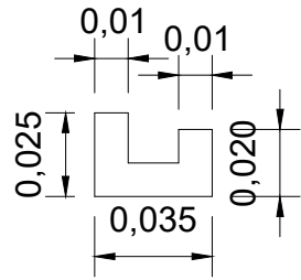
ELEVAÇÃO LATERAL
