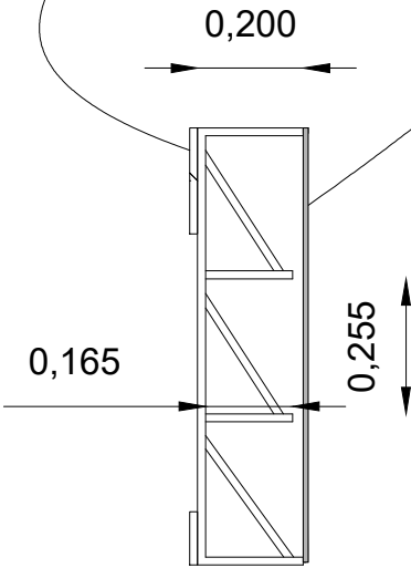
corte
