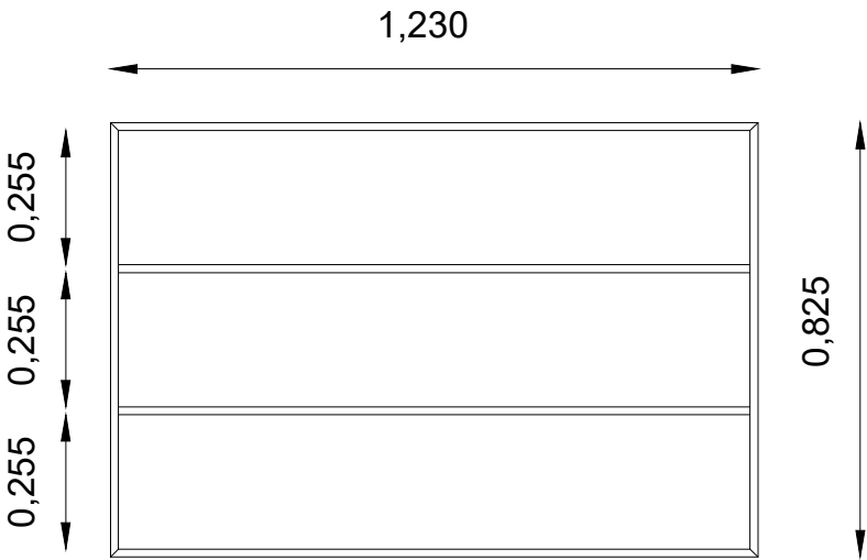
elevação frontal
