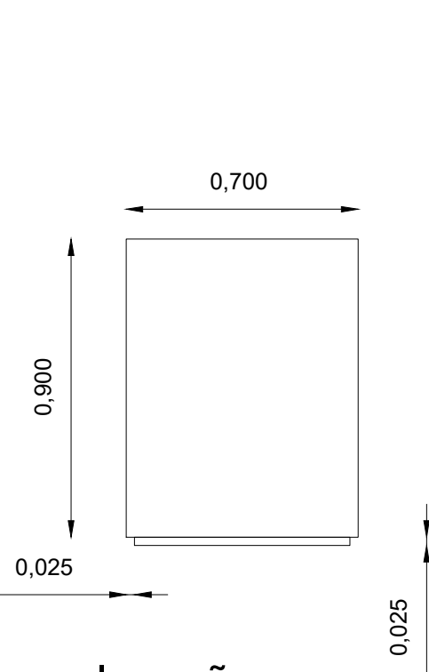
elevação
