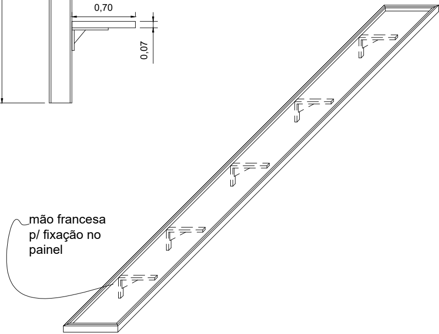
Perspectiva
