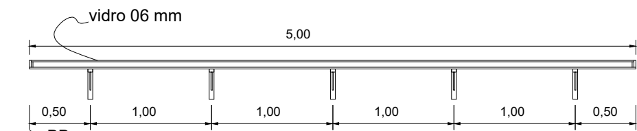
corte BB
