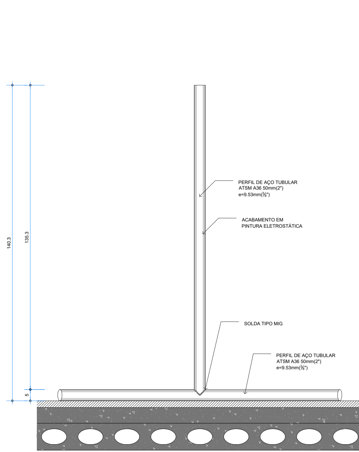
ELEVACÃO 1:10
