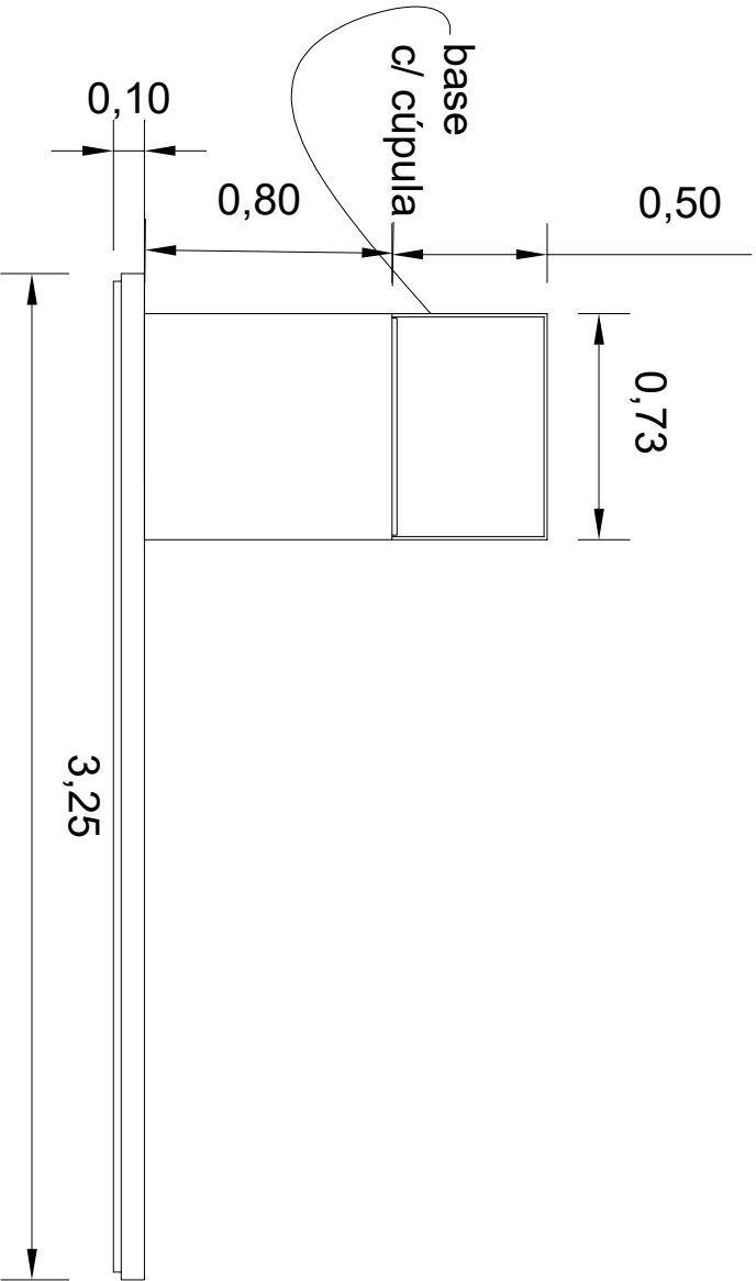
elevação lateral
