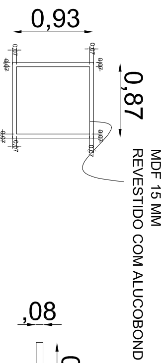
PLANTA
