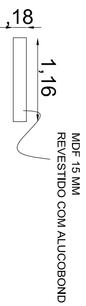
VISTA LATERAL
