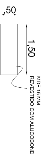
PLANTA
