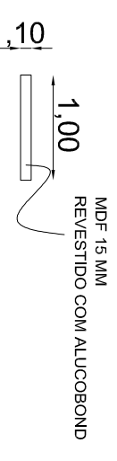
VISTA LATERAL
