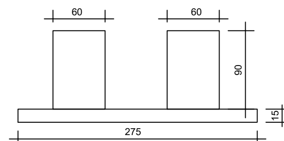
elevação
