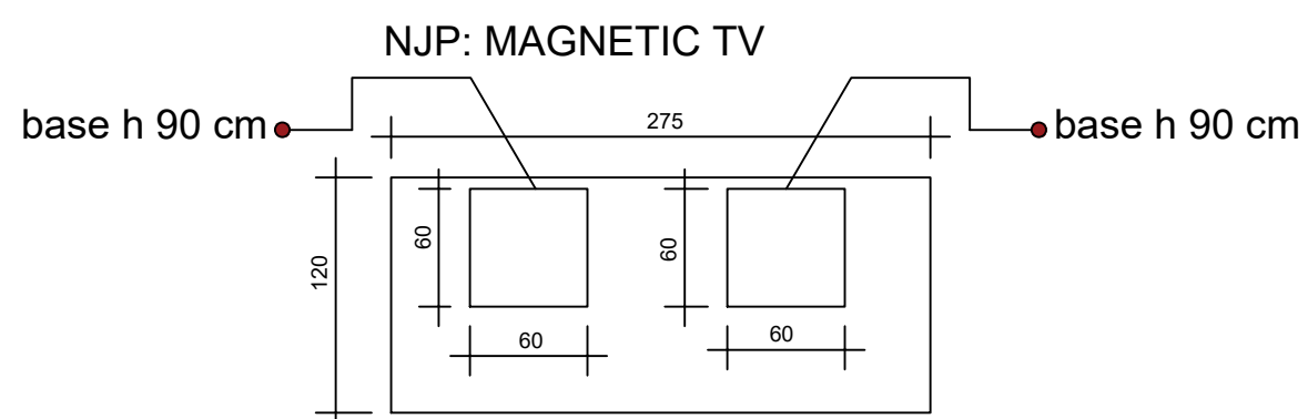
planta
