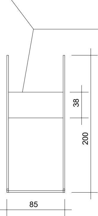
elevação frontal
