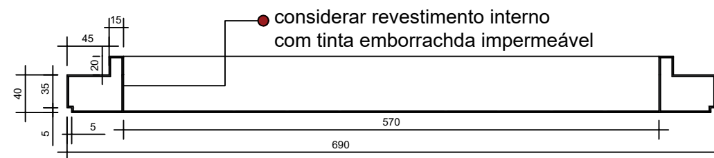
corte
