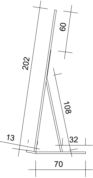
elevação lateral
