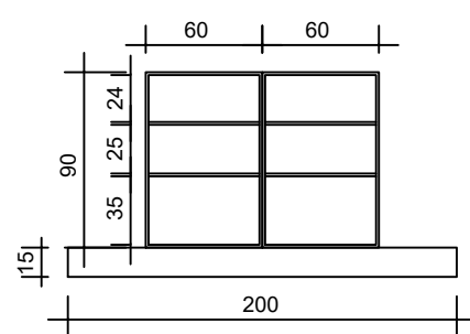
elevação frontal
