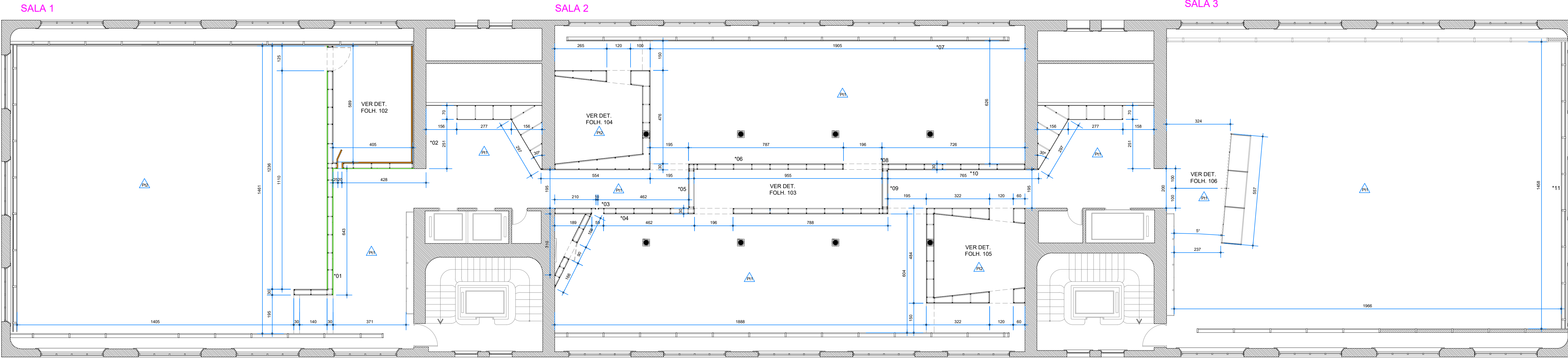
PLANTA EXPOGRAFIA + COTAS GERAIS 1:100
