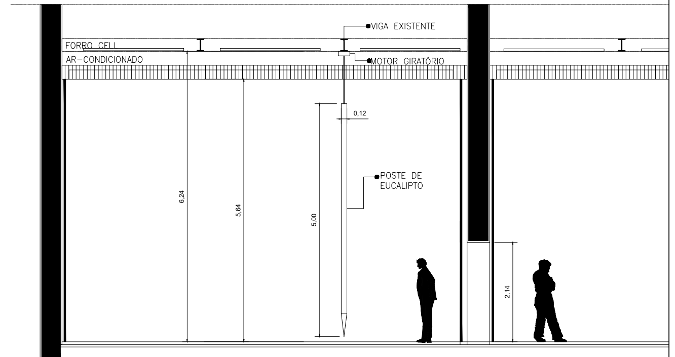
CORTE
