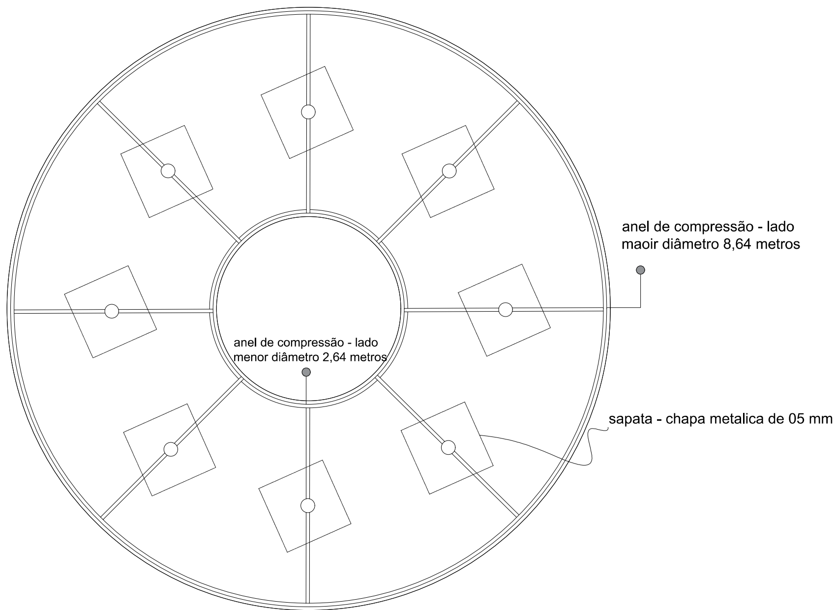
VISTA SUPERIOR
