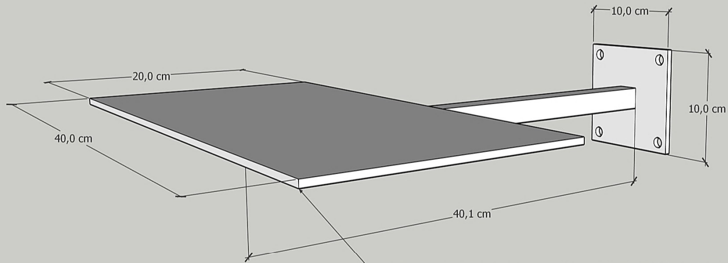
PRATELEIRA METALICA - CHAPA DE METAL 3MM/ HASTE METALON 2,5 X 2,5 CM/ SAPATA COM 4 FUROS COR CHOCOLATE - SUVINIL FOSCO
