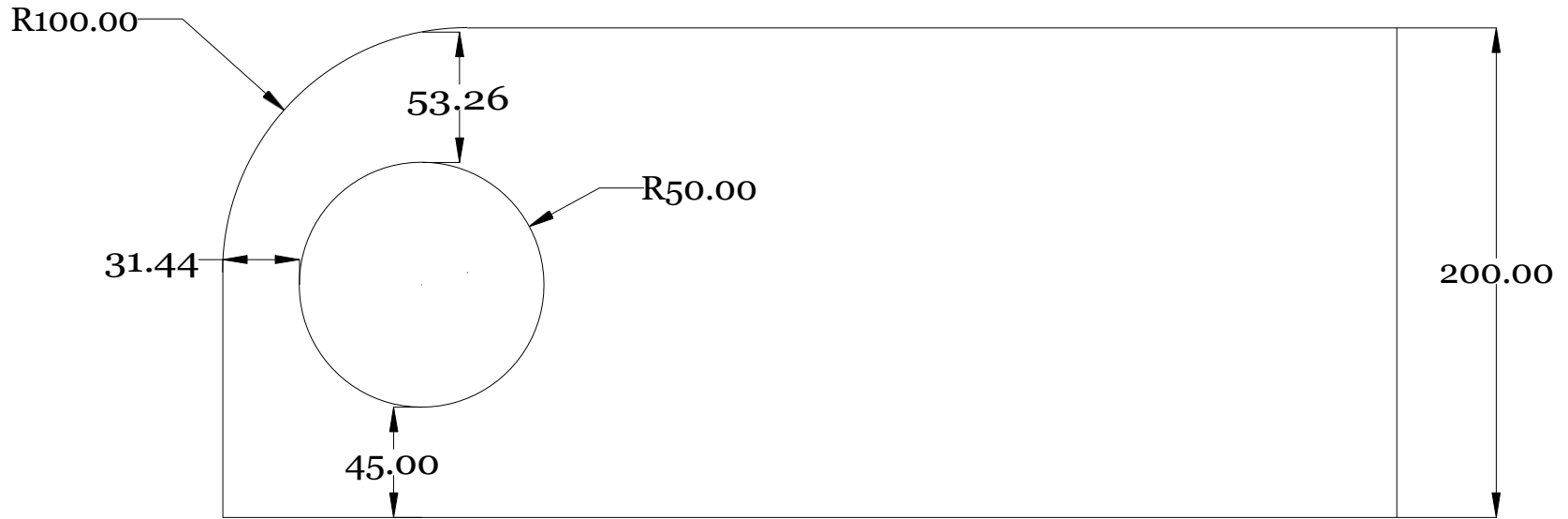
DETALHE PAINÉL - FRONTAL
