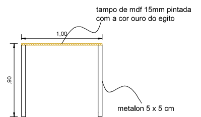
vista lateral
