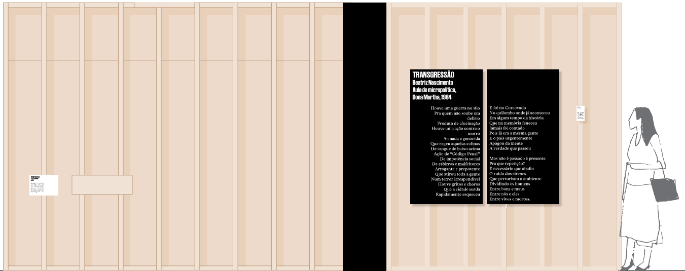
Placa com leitura em Braille, PS na cor preta (lateral visível) 3mm espessura. Fixação com placa de PS dobrada na angulação 45°.
