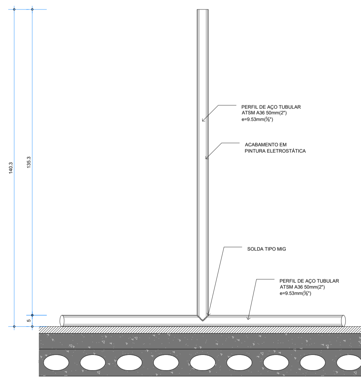
ELEVACÃO 1:10
