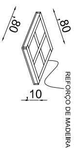
PERSPECTIVA
